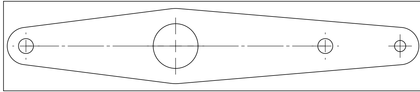
E16-3120 - 1 EA. SCISSOR BEAM, PILOT
